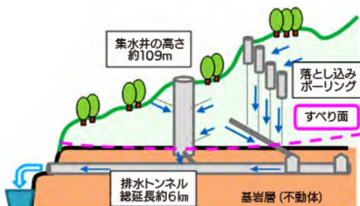
【地下水排水のイメージ図】
